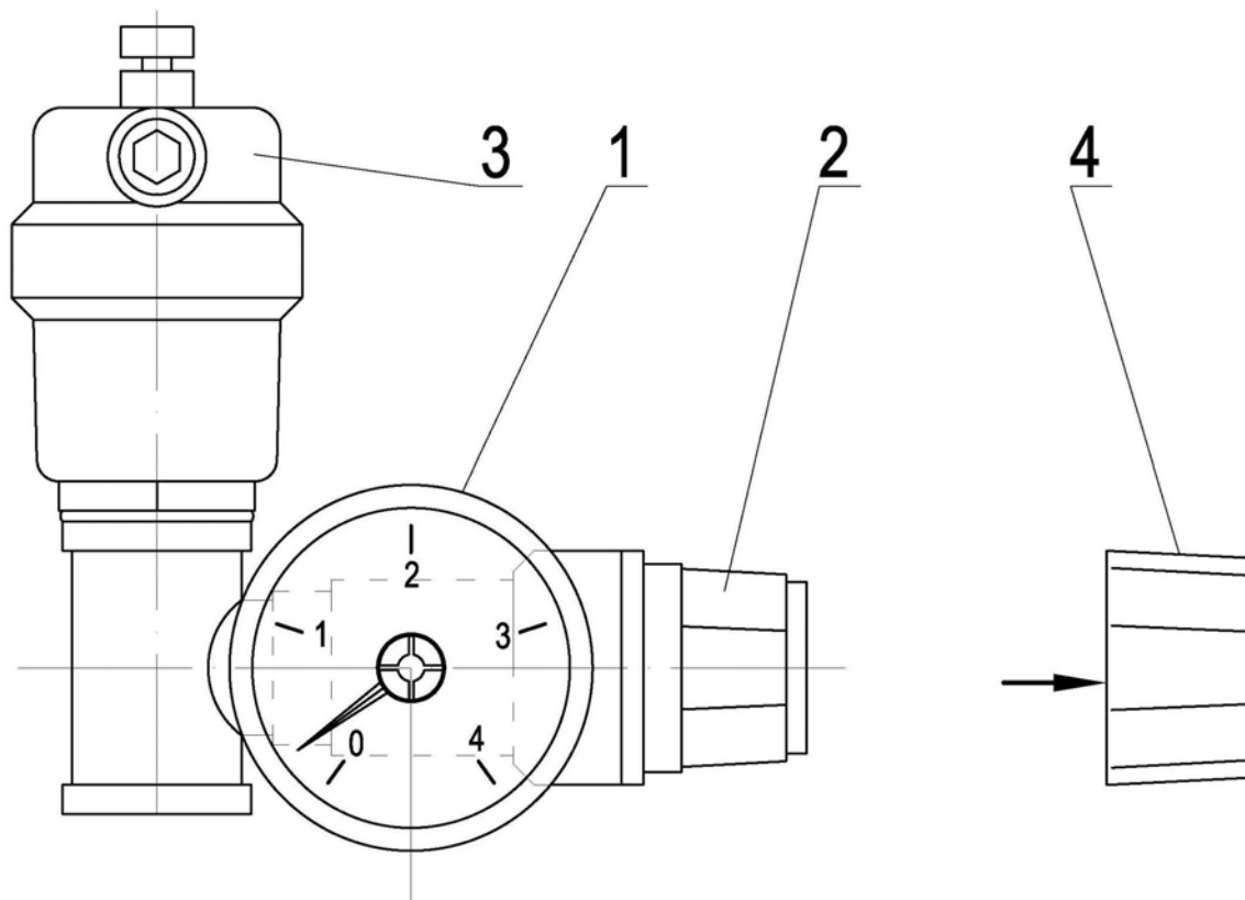
Рис.2 Предохранительная сборка
